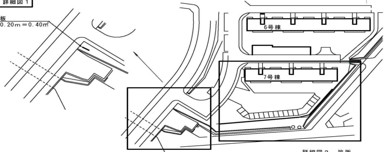
詳細図 1 箇所
