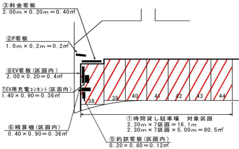
詳細図 1
