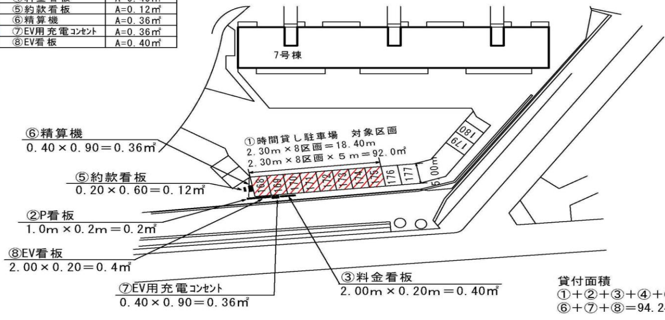
詳細図 2
