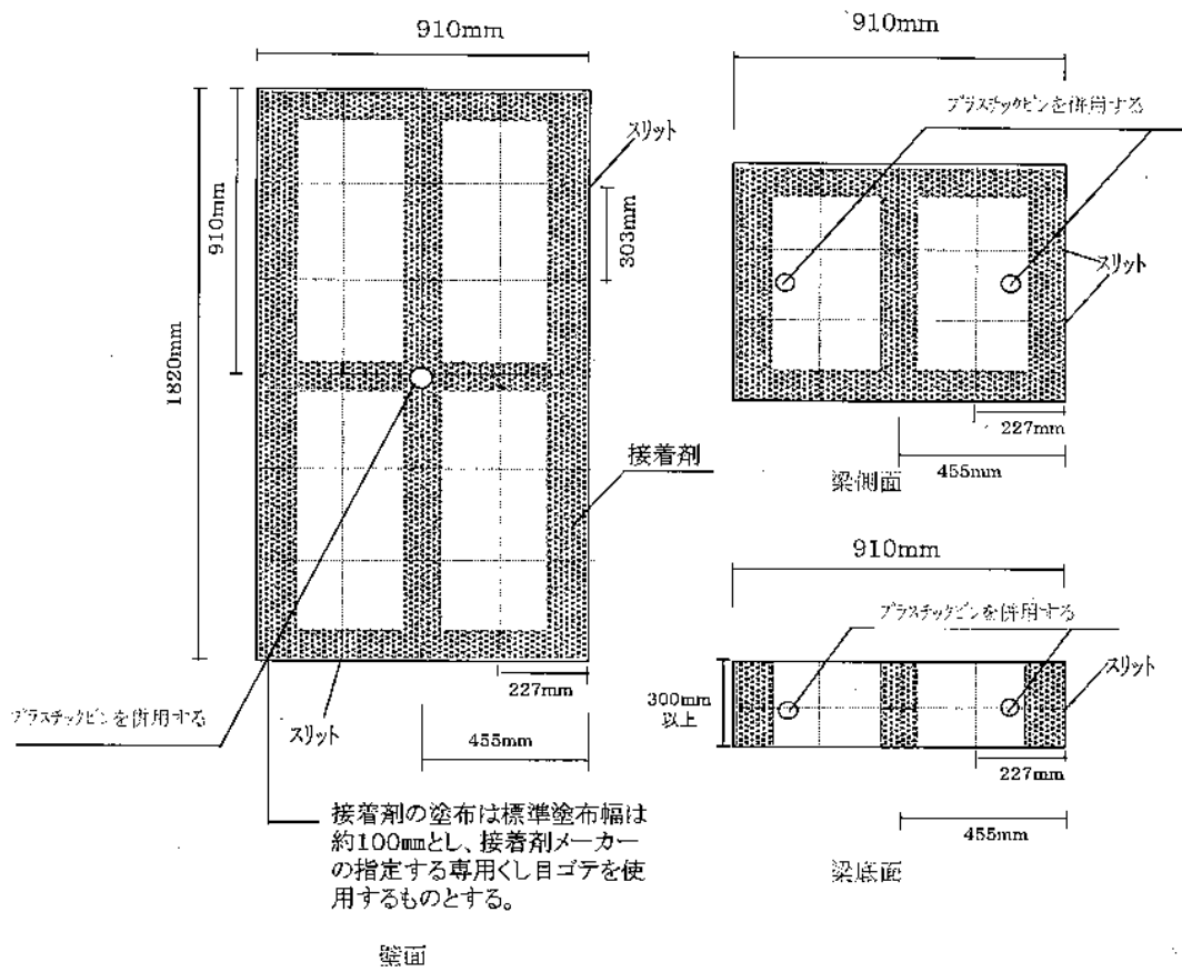
12.8.1 図 接着剤塗布、スリット及びプラスチックピンの標準位置図 (壁面、 はり 梁側面及び幅 300mm 以上の はり 梁底面)
