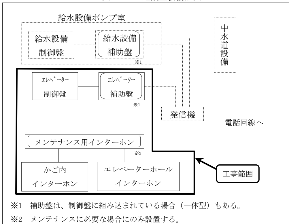
図9.9.1 遠隔監視構成図
