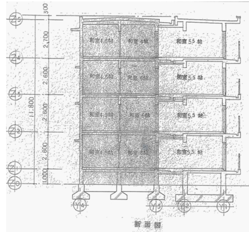
■南3・4・5・6号棟 断面図 (参考) Non Scale
