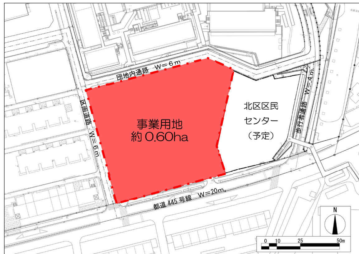
⑥将来位置図 S=1/1,500
